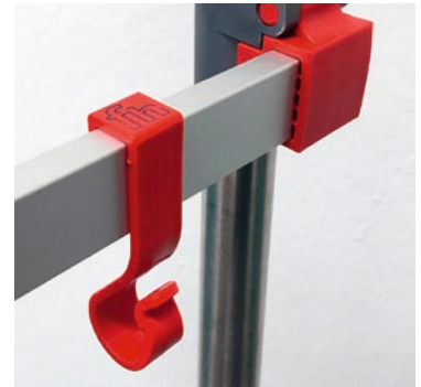
Instrumentenhaken zur Montage an Reling oder Edelstahlrohr
