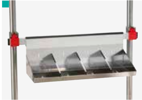
Stainless steel shelf with 3 removable dividers Estante de acero inox con 3 separadores extraíbles
